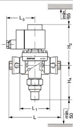
DEVSC10结构示意图
