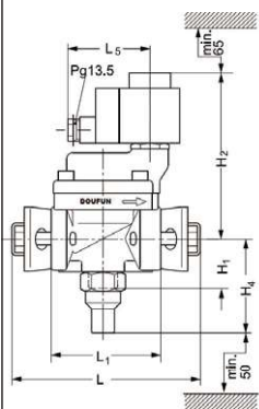
DEVSC25结构示意图
