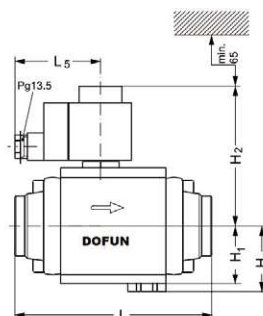
DEVSC25 DEVSC32 DEVSC40结构示意图
